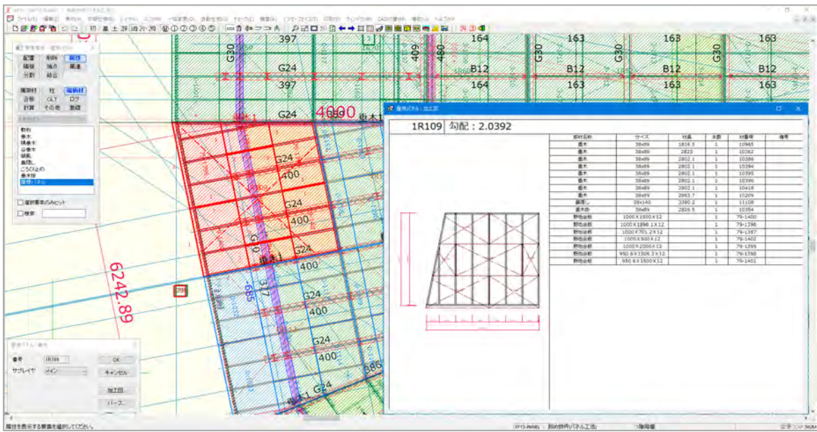
屋根パネル入力画面
